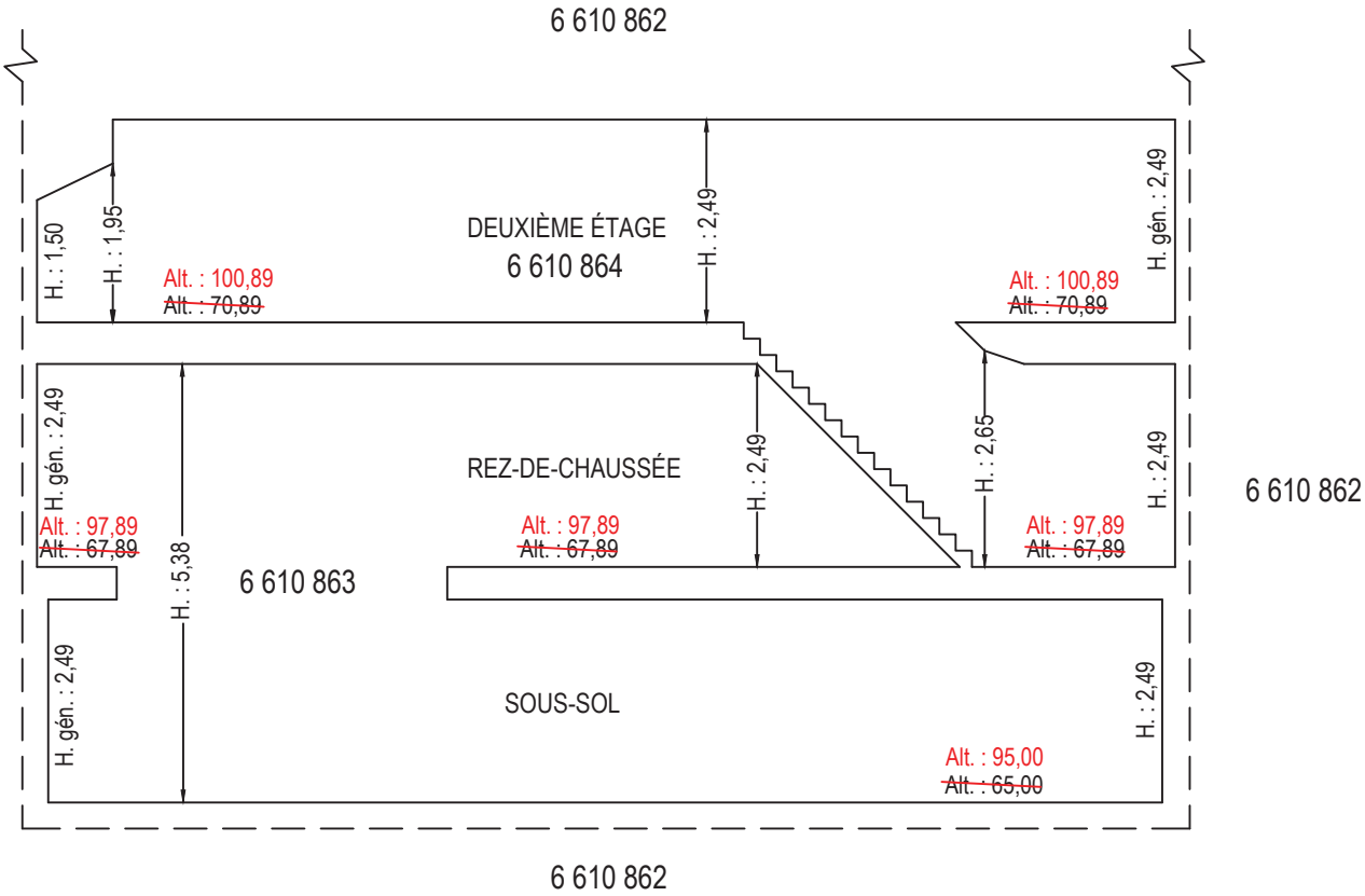
COUPE A-A
